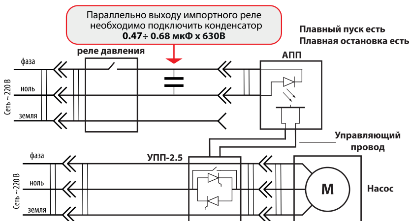
Схема 6. Подключение УПП к импортным реле давления с помощью адаптера плавного пуска АПП
