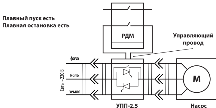
Схема 5. Подключение УПП-2.5 к механическому реле давления типа РДМ с помощью управляющего провода
